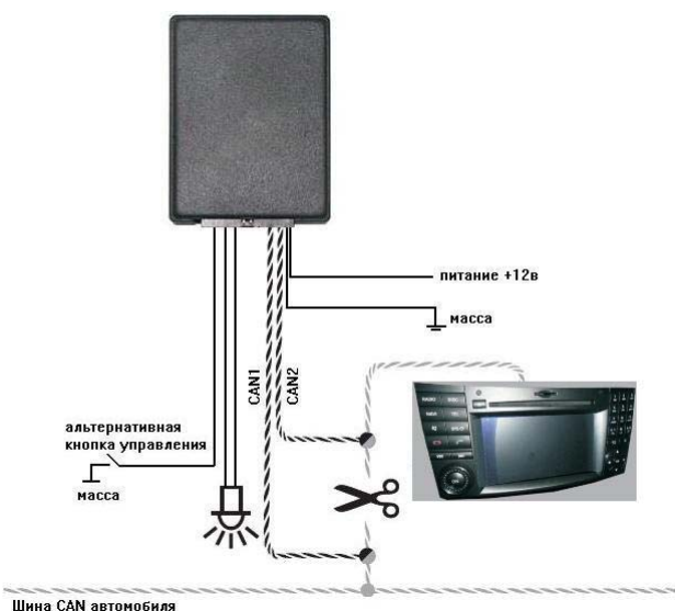
Шина CAN автомобиля
