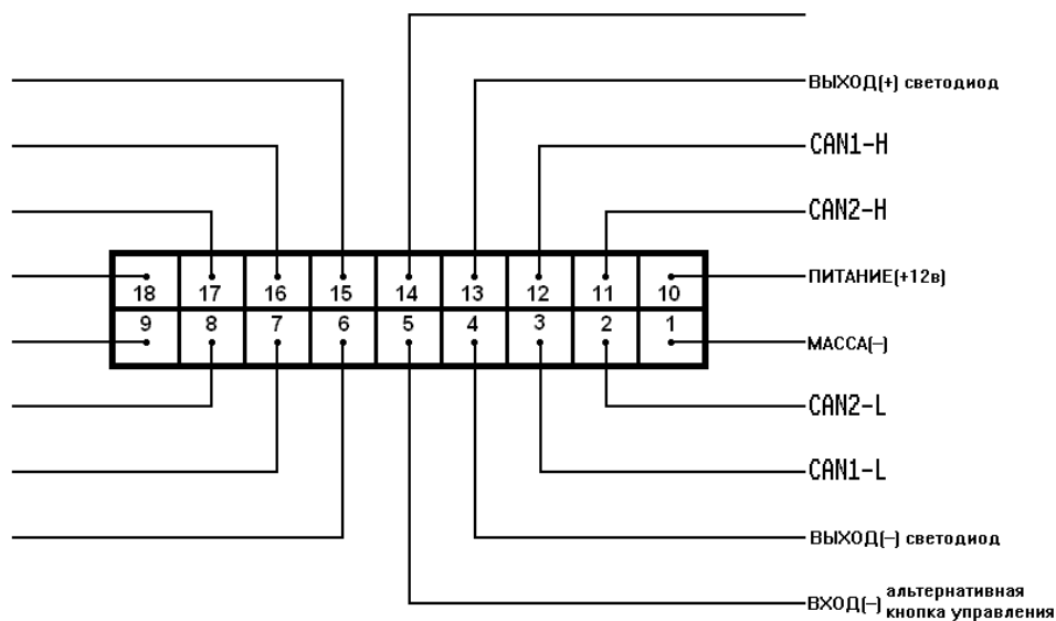
Назначение выводов модуля.
